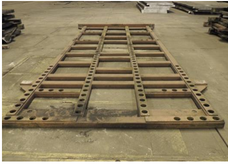
Рис. 11 Рама «ВО ПГП» (P-1)
